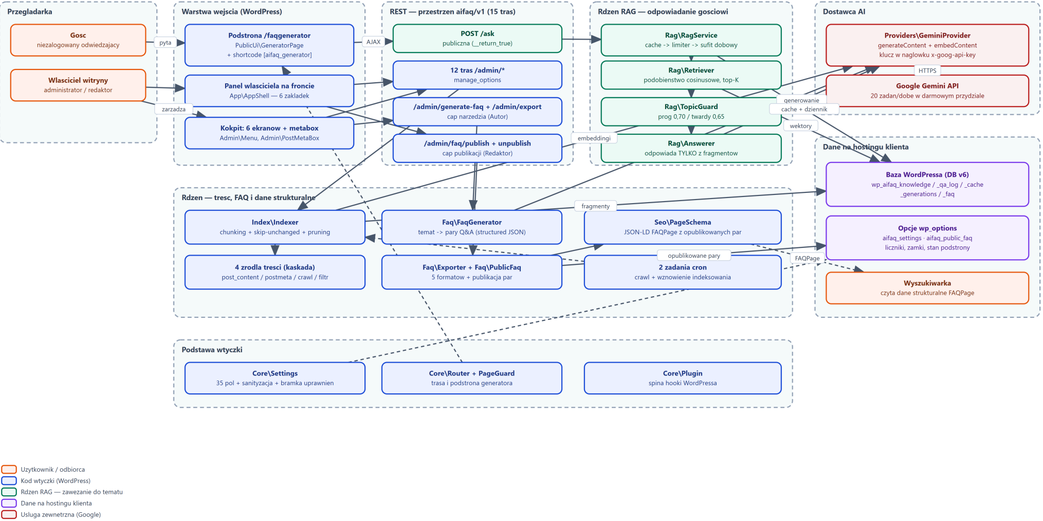
Architektura wykonawcza AI FAQ Generator · pełna skala w pliku źródłowym schematy/01-architektura-runtime.drawio
